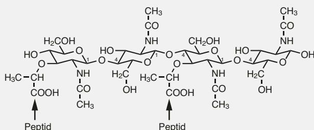
Verknüpfung von N -Acetylmuraminsäure (M) und N -Acetylglucosamin (A) im Murein
