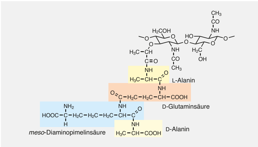
● Abb. 1.12 Mucopetideinheit (Peptidoglykan) aus einer Bakterienzellwand
