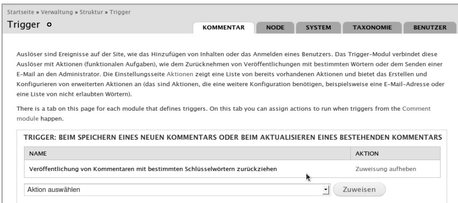
Bild 5.14: Aktion und Ereignis verknüpfen
